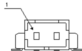
53261-0271 : molex
